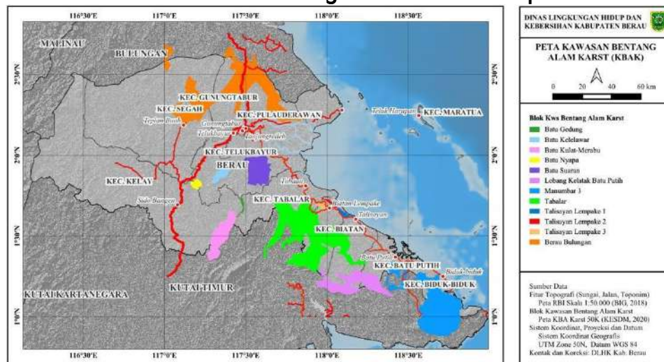
Gambar 2.4 Peta Indikatif Kawasan Bentang Alam Karst di Kabupaten Berau
